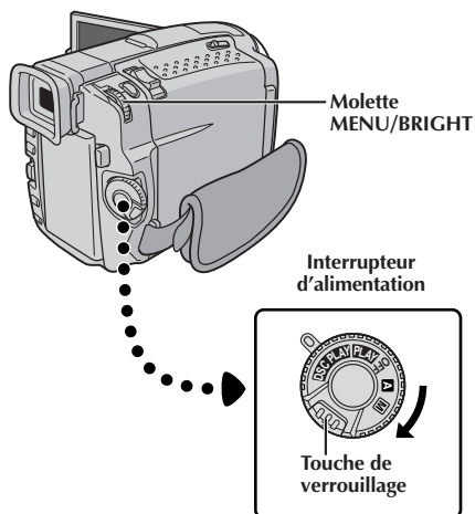
Affichage
